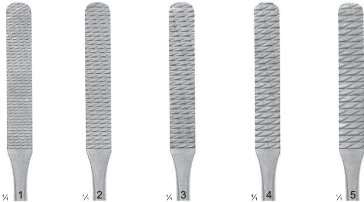
¼ 1 ¼ 2 ¼ 3 ¼ 4 ¼ 5 57-100-01 57-100-02 57-100-03 57-100-04 57-100-05 12 Teeth 12 Zähne 12 Dientes 12 Dents 12 Denti 14 Teeth 14 Zähne 14 Dientes 14 Dents 14 Denti 16 Teeth 16 Zähne 16 Dientes 16 Dents 16 Denti 20 Teeth 20 Zähne 20 Dientes 20 Dents 20 Denti 24 Teeth 24 Zähne 24 Dientes 24 Dents 24 Denti
